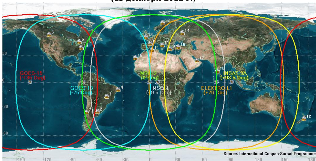
Рисунок 6: Зоны видимости геостационарных спутников и ГЕОСПОИ (15 декабря 2012 г.)
