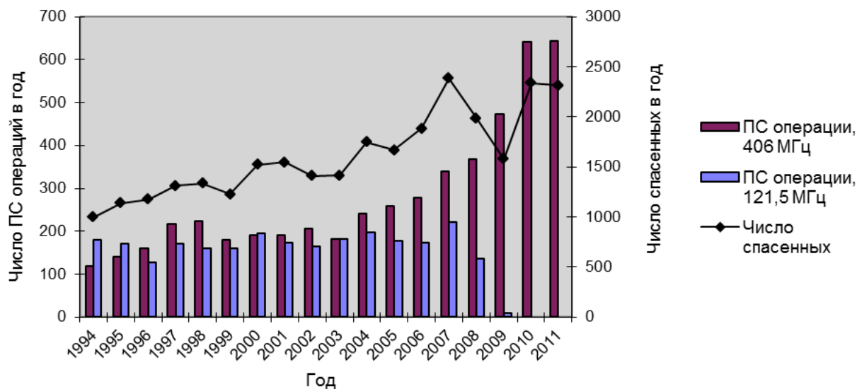
Рисунок 4: Число ПСО и число спасенных в ПСО, использовавших данные Системы Коспас-Сарсат (январь 1994 г. - декабрь 2011 г.)
