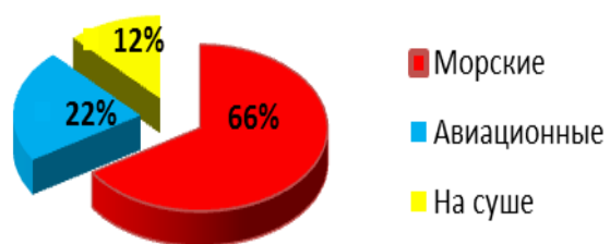
Рисунок 3: Спасенные по типу ПСО, использовавших данные Системы Коспас-Сарсат (январь - декабрь 2011 г.)
