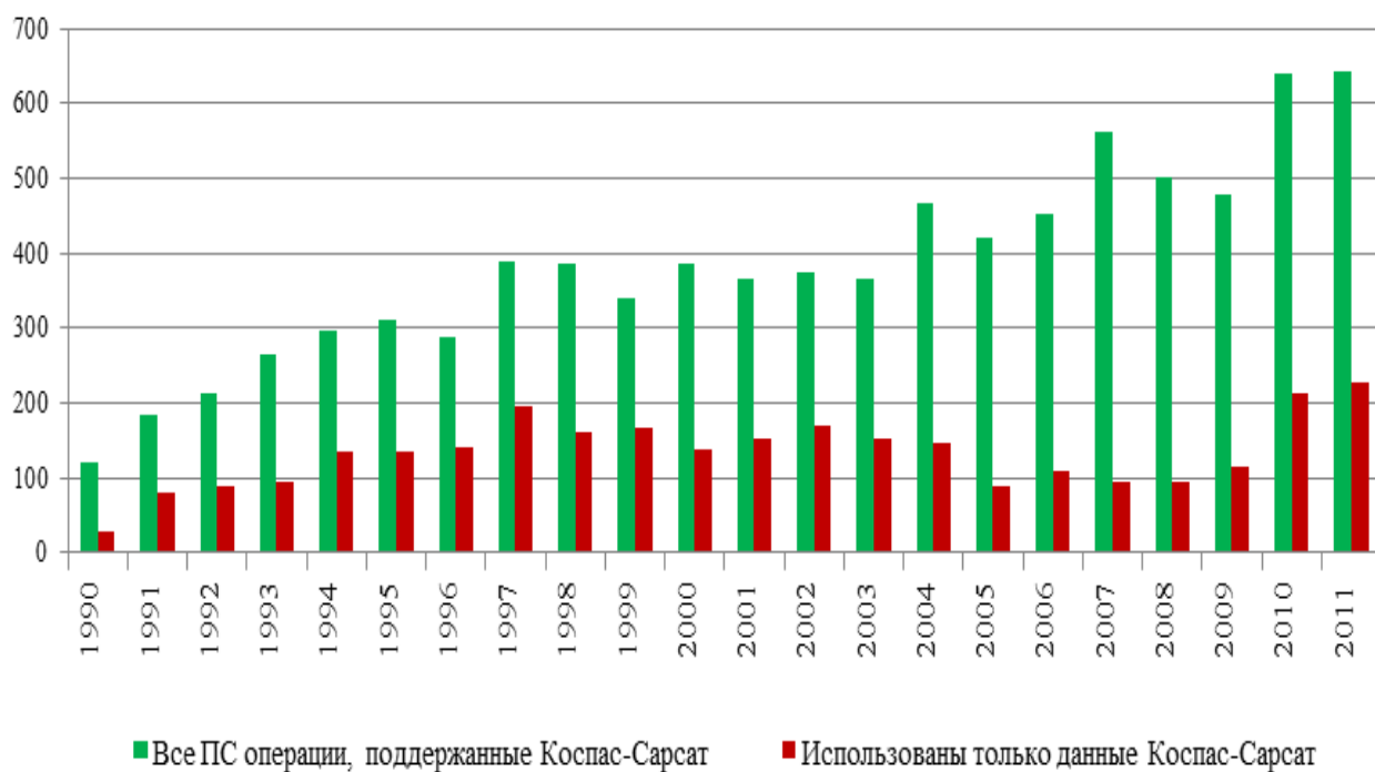
Рисунок 5: Число ПСО, в которых использовались данные Системы Коспас-Сарсат, и число ПСО, в которых были использованы только данные Система Коспас-Сарсат (январь 1990 - декабрь 2011 г.)
