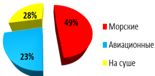
Рисунок 2: Тип ПСО, использовавших данные Системы Коспас-Сарсат (январь - декабрь 2011 г.)
